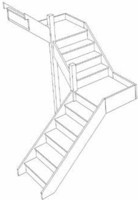
Stair-S5QL3QL2N-LH
