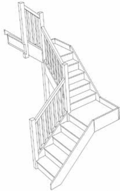
Stair-S4QL4QL2N-LH-HR
